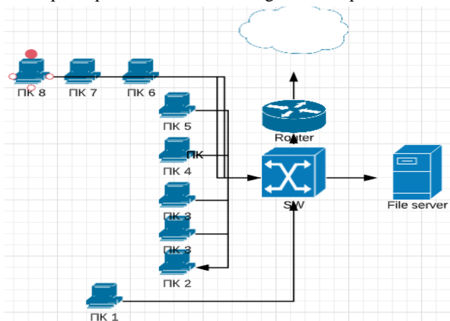
Рисунок 1 - Схема підключення комп'ютерів в мережу
